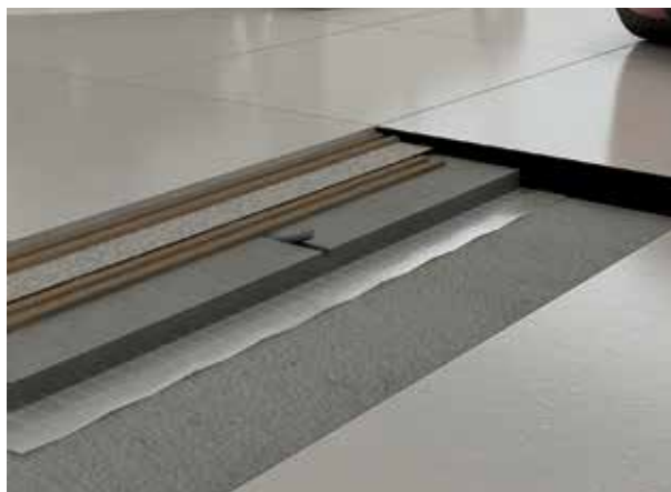
Skladba systému MAPETEX: Keraquick + MapeTex Vlies,
